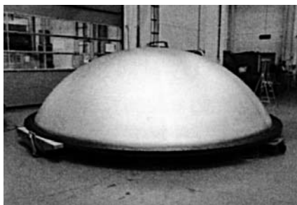
Днище корпуса космического аппарата, сваренного трением.
