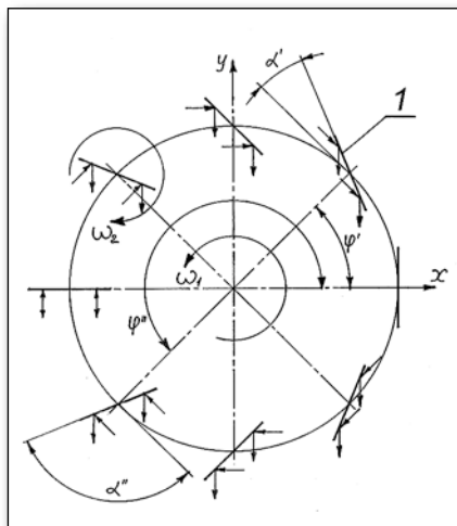
Рис.1. Схема работы планетарной лопаточной машины.
