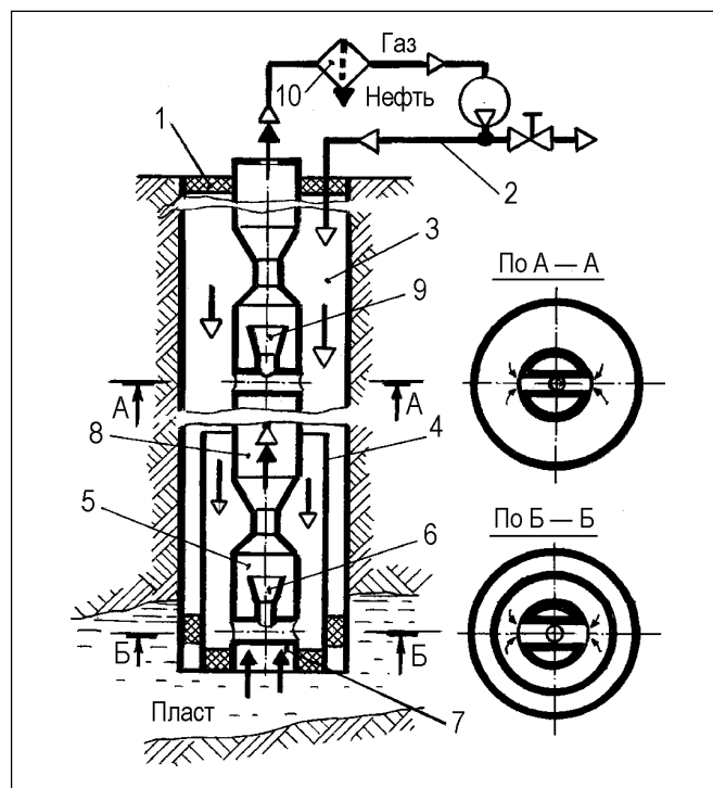
Газлифтная установка.
