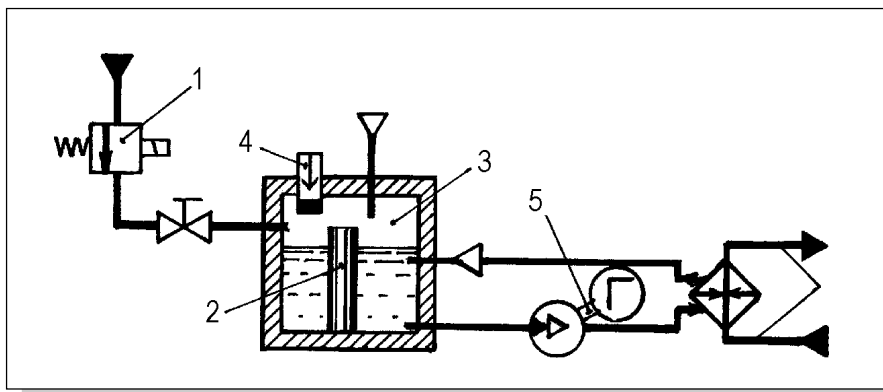
Энергетическая установка.
