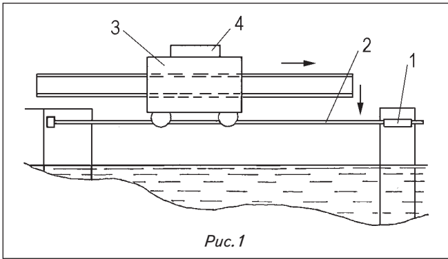
Струнный «монтажник» мостовых пролетов.
