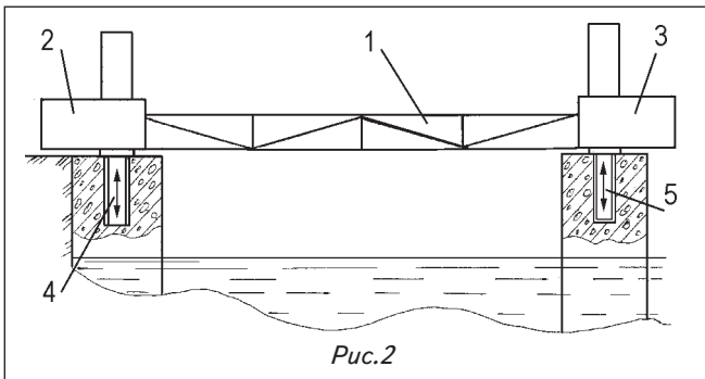
Схема мобильной кран-балки.
