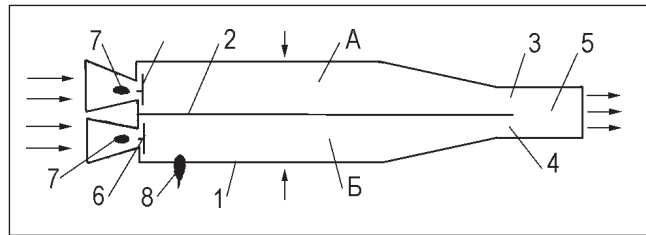
Схема простого и долговечного реактивного двигателя.
