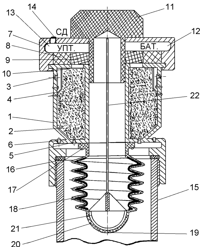
Схема устройства заправки «Приз-6».
