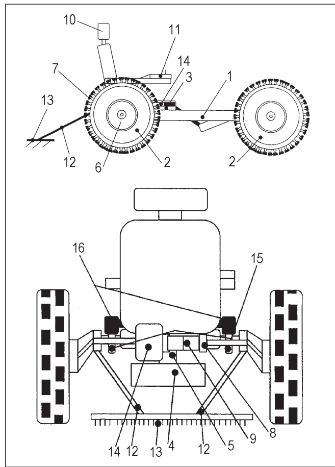
Схема инвалидной коляски, столь же надежно катающейся по лестницам, как и по гладкому асфальту тротуаров.
