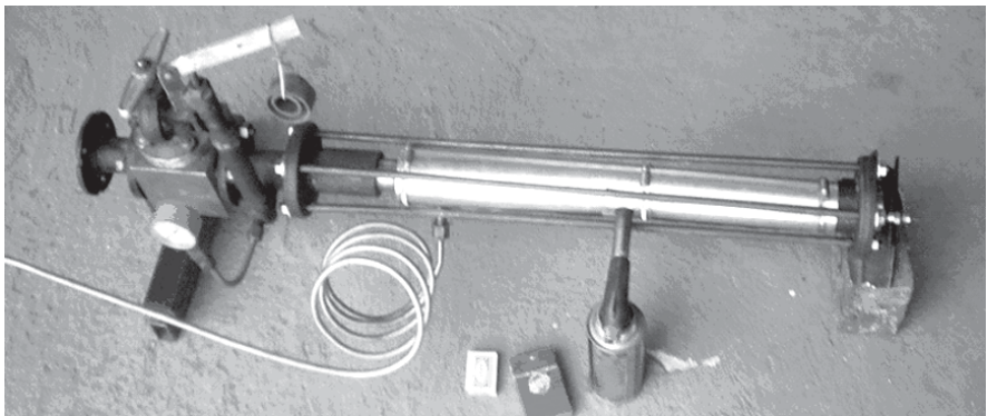
Опытная реакционная камера для термоллиза азотного топлива постоянного давления.
